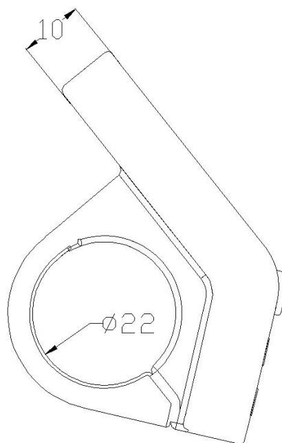
仪表主体外形尺寸
