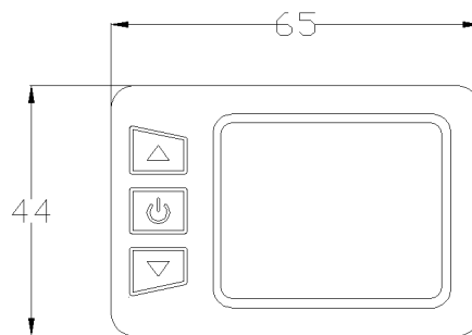
仪表主体外形尺寸
