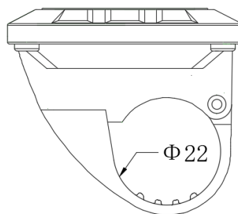
仪表主体外形尺寸
