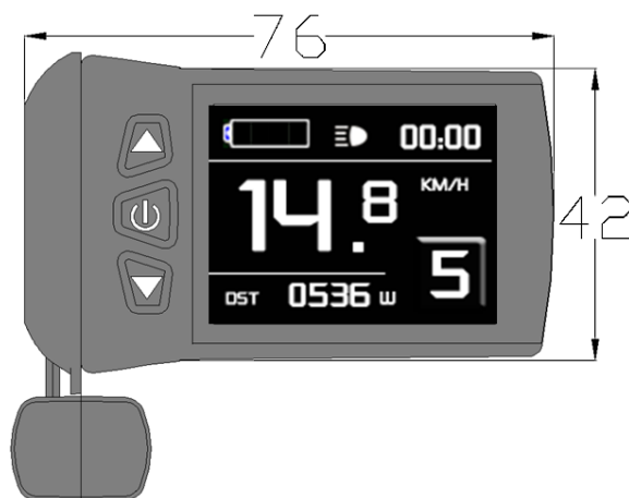
仪表主体外形尺寸
