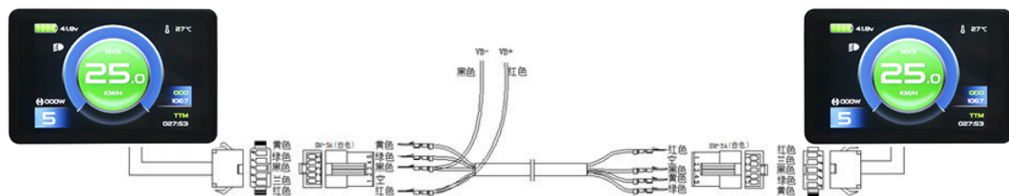
仪表参数复制连线图
