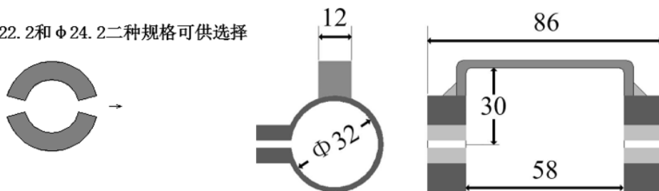
双支架安装尺寸
